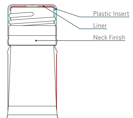
Stelvin® Lux / Stelvin® Lux+
